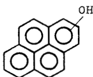
pyrenol
